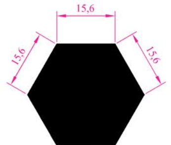
Profil No : 1815 Ağırlık : 1,084 kg/m
