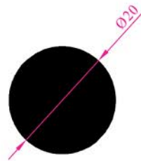
Profil No : 1821 Ağırlık : 0,880 kg/m
