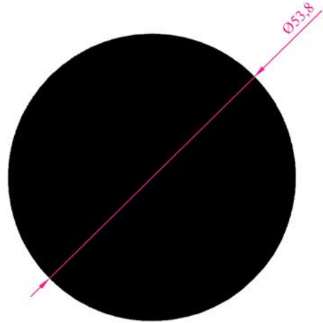
Profil N o : 1811 Ag ırık : 6,365 kg/m
