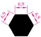
Profil No : 1831 Ağırlık : 0,338 kg/m
