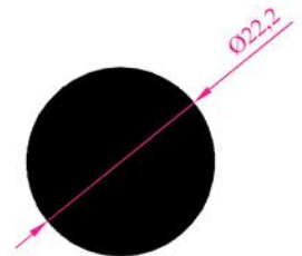
Profil No : 1815 Ağırlık : 1,084 kg/m
