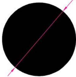
Profil N o :1810 Ag ırık :2,179 kg/m
