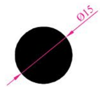
Profil No : 1819 Ağırlık : 0,495 kg/m
