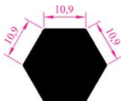
Profil No : 1832 Ağırlık : 0,847 kg/m
