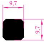
Profil No : 1848 Ağırlık : 0,249 kg/m
