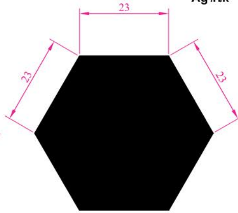
Profil N o :1837 Ag ırık :3,755 kg/m
