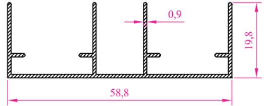
Profil N o :2561 Ag ırık 0,361 kg/m
