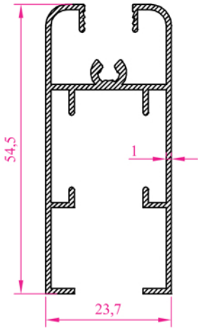
Profil N o :2233 Ağırlık 0,530 kg/m
