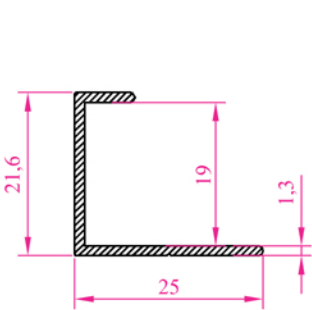
Profil N o :2207 Ag ırık 0,182 kg/m
