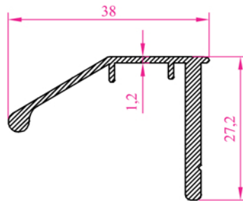
Profil N o :2629 Ag.ırlık 0,387 kg/m
