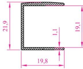
Profil N o :2205 Ag ırık 0,197 kg/m
