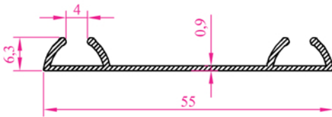
Profil N o :2589 Ag ırık 0,217 kg/m
