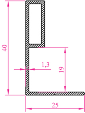
Profil N o : 2213 Ag ırık 0,331 kg/m
