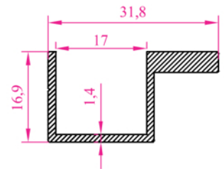
Profil N o :2596 Ag.ırlık 0,319 kg/m
