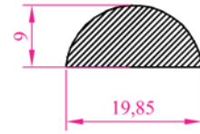
Profil N o :2690 Ag.ırlık 0,372 kg/m
