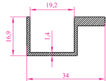
Profil N o : 2224 Ag ırık 0,327 kg/m
