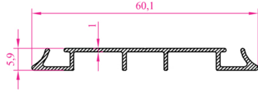
Profil N o :2232 Ağırlık 0,260 kg/m
