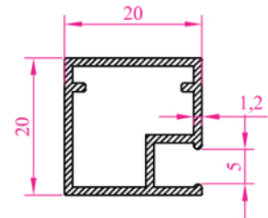
Profil N o : 2227 Ag ırık 0,283 kg/m
