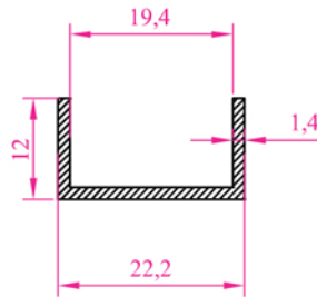
Profil N o : 2223 Ag ırık 0,165 kg/m
