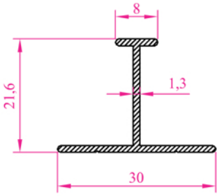
Profil N o :2201 Ag ırık 0,198 kg/m
