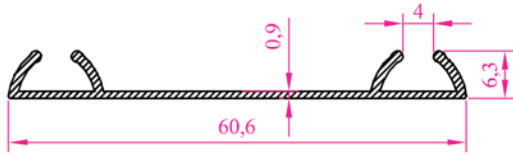
Profil N o :2560 Ag ırık 0,231 kg/m
