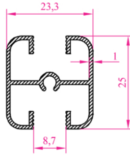
Profil N o : 2217 Ag ırık 0,304 kg/m
