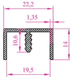
Profil N o :2211 Ag ırık 0,239 kg/m
