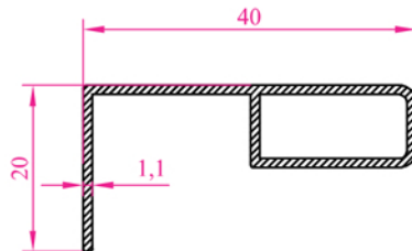
Profil N o : 5290 Ag ırık 0,277 kg/m
