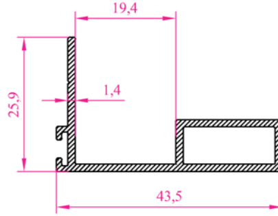
Profil N o : 2214 Ag ırık 0,403 kg/m
