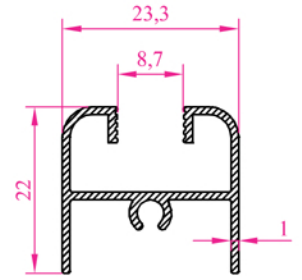
Profil N o : 2218 Ag ırık 0,248 kg/m
