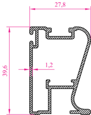
Profil N o : 2225 Ag ırık 0,565 kg/m
