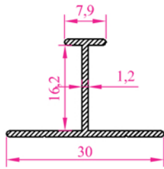
Profil N o : 5012 Ag ırık 0,173 kg/m
