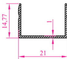
Profil N o :2624 Ag.ırlık 0,226 kg/m
