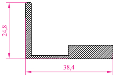
Profil N o : 2714 Ag ırık 0,547 kg/m
