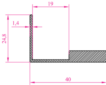
Profil N o : 2222 Ag ırık 0,484 kg/m
