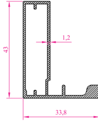
Profil N o :2240 Ag ırık 0,488 kg/m
