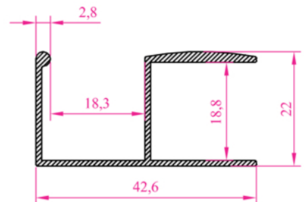
Profil N o :2212 Ag ırık 0,358 kg/m
