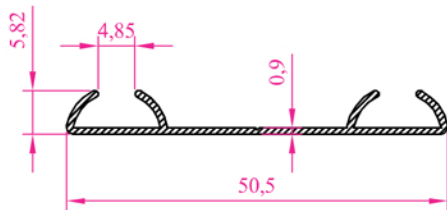
Profil N o :2564 Ag ırık 0,182 kg/m
