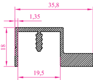
Profil N o :2210 Ag ırık 0,511 kg/m
