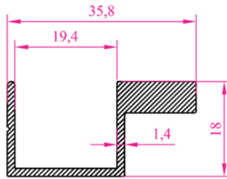
Profil N o :2208 Ag ırık 0,435 kg/m
