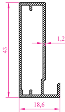
Profil N o :2237 Ağırlık 0,371 kg/m
