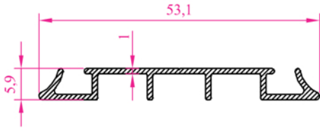
Profil N o :2231 Ağırlık 0,241 kg/m
