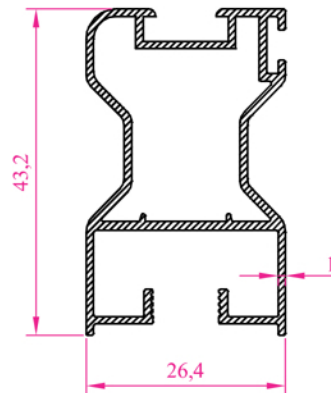
Profil N o : 2220 Ag ırık 0,510 kg/m
