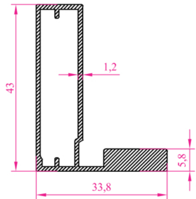
Profil N o :2238 Ağırlık 0,608 kg/m
