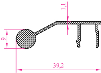
Profil N o :2621 Ag.ırlık 0,335 kg/m
