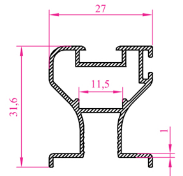
Profil N o : 2221 Ag ırık 0,378 kg/m
