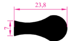
Profil N o : 5366 Ag ırık 0,488 kg/m
