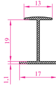
Profil N o :2203 Ag ırık 0,146 kg/m
