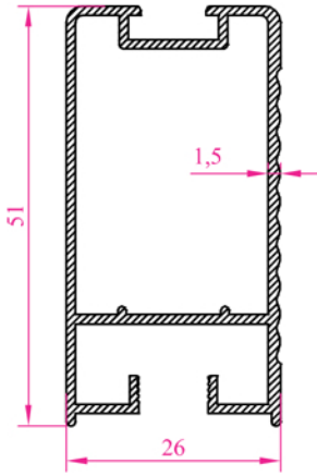
Profil N o :2234 Ağırlık 0,578 kg/m
