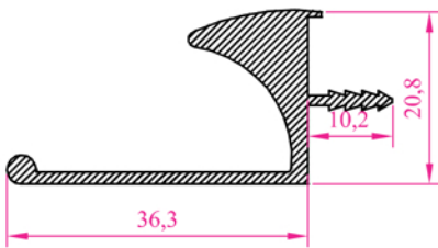
Profil N o : 5019 Ag ırık 0,531 kg/m
