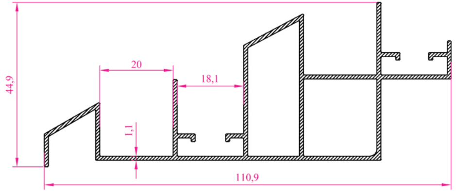
Profil N o : 2736 Ag ırık 1,005 kg/m
