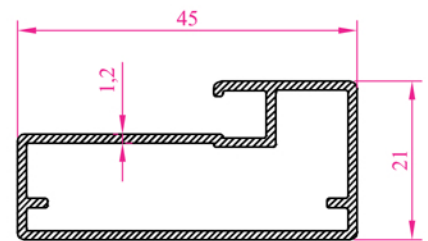
Profil N o : 2230 Ag ırık 0,461 kg/m
