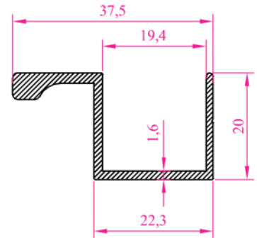
Profil N o :2206 Ag ırık 0,370 kg/m
