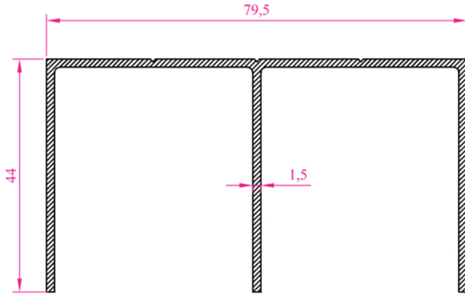
Profil N o :2611 Ag.ırlık 0,842 kg/m
