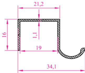
Profil N o :2204 Ag ırık 0,204 kg/m
