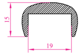
Profil N o : 5232 Ag ırık 0,374 kg/m
