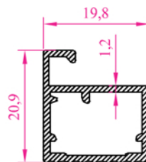
Profil N o : 2229 Ag ırık 0,271 kg/m
