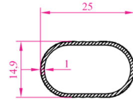
Profil N o :2566 Ag ırık 0,162 kg/m
