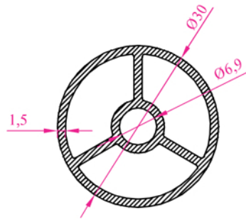
Profil N o : 5112 Ag ırık 0,577 kg/m
