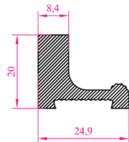
Profil N o :2597 Ag.ırlık 0,608 kg/m
