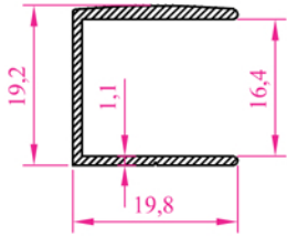
Profil N o :2239 Ag ırık 0,189 kg/m
