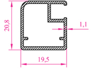
Profil N o : 2215 Ag ırık 0,269 kg/m
