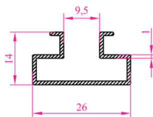
Profil N o :2623 Ag.ırlık 0,194 kg/m
