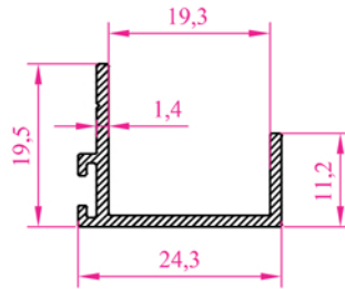
Profil N o :2202 Ag ırık 0,211 kg/m
