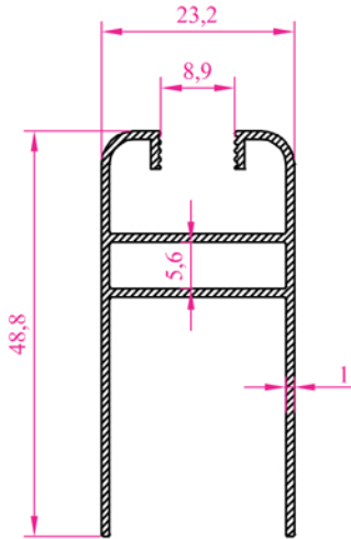
Profil N o : 2216 Ag ırık 0,425 kg/m
