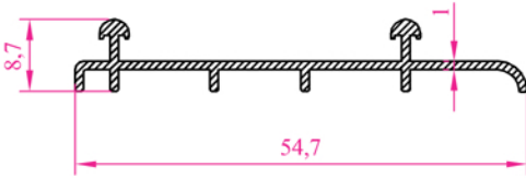
Profil N o : 2219 Ag ırık 0,236 kg/m
