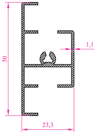
Profil N o :2236 Ağırlık 0,450 kg/m
