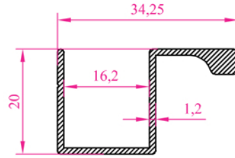
Profil N o : 5013 Ag ırık 0,290 kg/m
