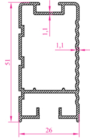
Profil N o :2235 Ağırlık 0,572 kg/m
