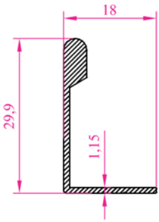
Profil N o : 5006 Ag ırık 0,217 kg/m
