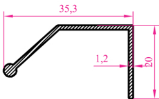
Profil N o : 5289 Ag ırık 0,205 kg/m
