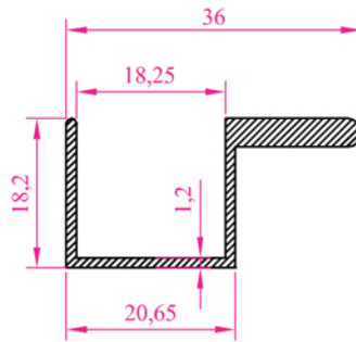
Profil N o : 2226 Ag ırık 0,319 kg/m
