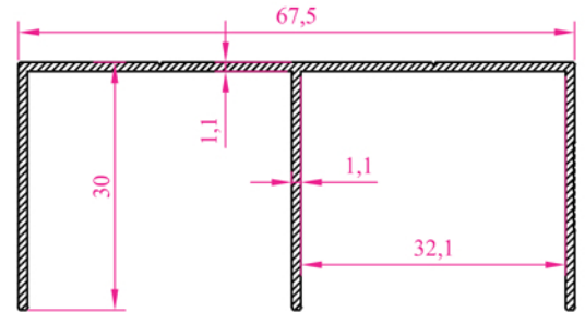
Profil N o :2209 Ag ırık 0,456 kg/m
