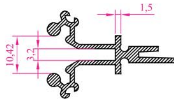
Profil N o : 2617 Ag ırık : 0,395 kg/m
