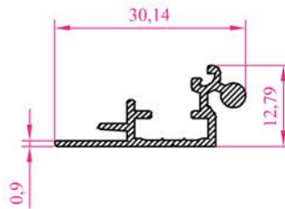
Profil N o : 2255 Ag ırık : 0,201 kg/m
