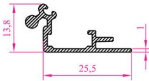
Profil N o : 2618 Ag ırık : 0,205 kg/m
