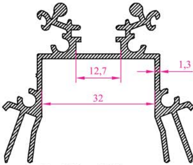
Profil N o : 2616 Ag ırık : 0,881 kg/m
