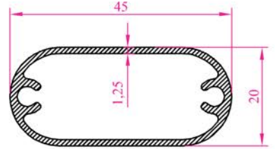
Profil N o : 2253 Ag ırık : 0,463 kg/m
