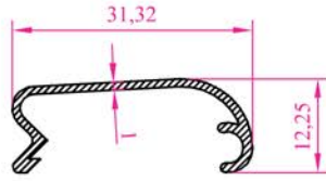
Profil N o : 2251 Ag ırık : 0,167 kg/m
