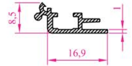
Profil N o : 2619 Ag ırık : 0,122 kg/m
