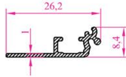
Profil N o : 2252 Ag ırık : 0,124 kg/m
