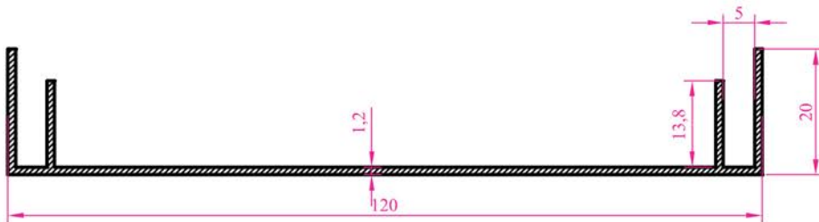
Profil N o : 2602 Ag ırık : 0,622 kg/m
