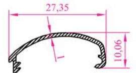
Profil N o : 2254 Ag ırık : 0,117 kg/m
