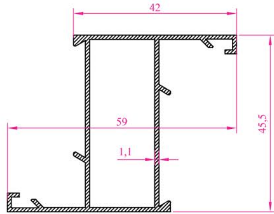
Profil N o :1005 Ag ırık :0,589 kg/m
