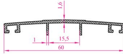
Profil N o : 2679 Ag ırık : 0,318 kg/m
