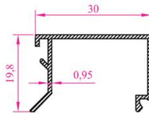
Profil No : 1006 Ag ırık : 0,205 kg/m
