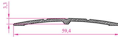
Profil N o : 2677 Ag ırık : 0,257 kg/m
