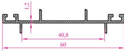
Profil N o : 2672 Ag ırık : 0,309 kg/m
