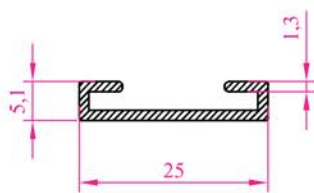
Profil No : 1021 Ag ırık : 0,145 kg/m
