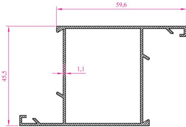
Profil N o :1002 Ag ırık :0,699 kg/m
