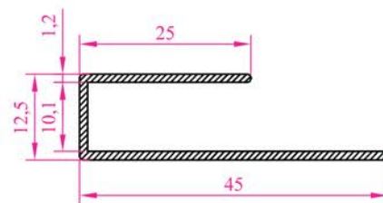
Profil N o :2674 Ag ırık 0,260 kg/m
