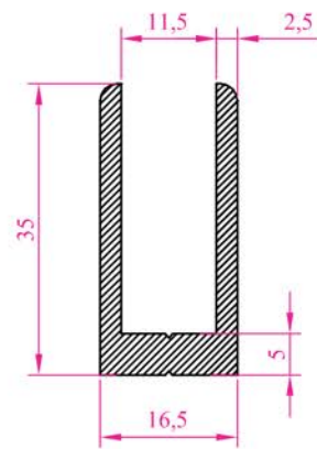
Profil No : 1017 Ag ırık : 0,624 kg/m
