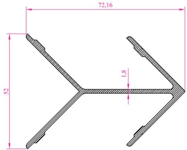
Profil No : 1012 Ag ırık : 0,973 kg/m
