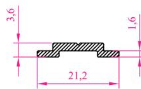
Profil No : 1022 Ag ırık : 0,119 kg/m
