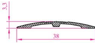
Profil N o : 2675 Ag ırık : 0,130 kg/m
