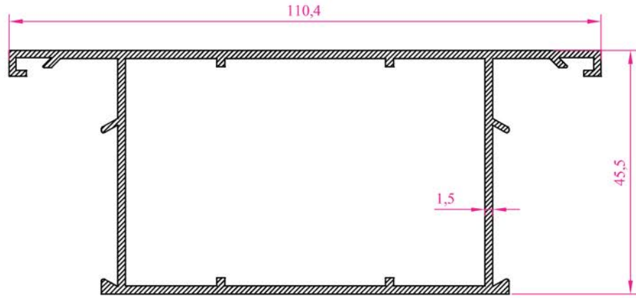
Profil No : 1009 Ag ırık : 1,203 kg/m
