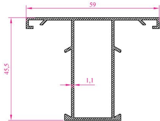
Profil N o :1004 Ag ırık :0,589 kg/m
