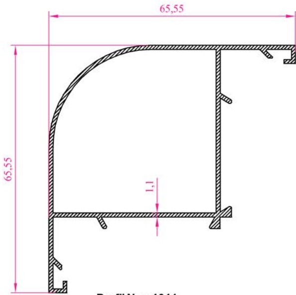
Profil No : 1011 Ag ırık : 0,719 kg/m
