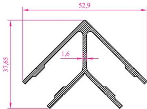
Profil No : 1013 Ag ırık : 0,661 kg/m
