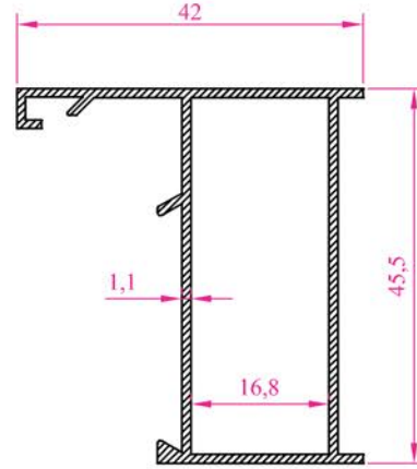
Profil N o :1003 Ag ırık :0,498 kg/m
