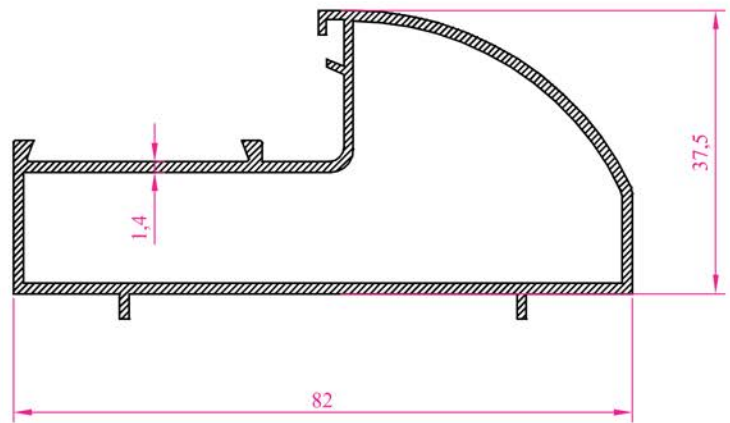
Profil N o :2628 Ag ırık 0,896 kg/m
