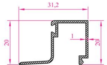
Profil No : 1007 Ag ırık : 0,211 kg/m
