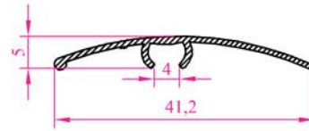
Profil N o : 2671 Ag ırık : 0,133 kg/m
