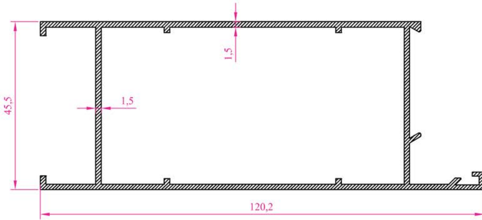
Profil N o : 1010 Ag ırık : 1,334 kg/m
