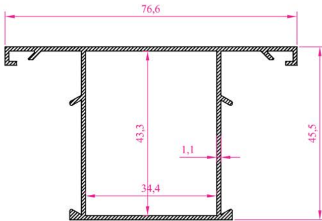
Profil N o :1001 Ag ırık :0,700 kg/m
