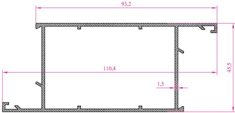
Profil N o : 1008 Ag ırık : 1,203 kg/m
