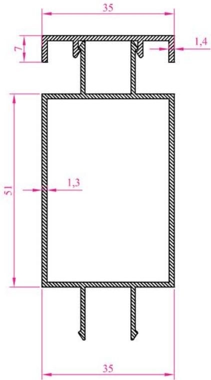
Profil N o :2600 Ag ırık 0,757 kg/m
