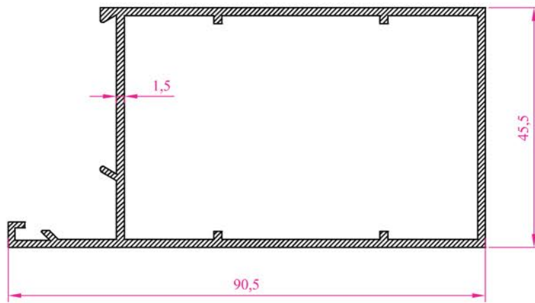
Profil No : 1018 Ag ırık : 1,072 kg/m
