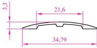
Profil N o : 2676 Ag ırık : 0,124kg/m
