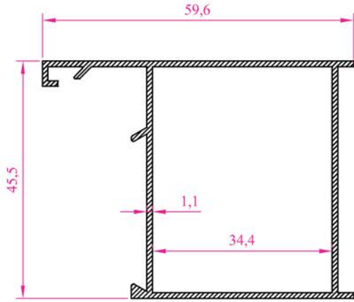
Profil N o :1000 Ag ırık :0,606 kg/m
