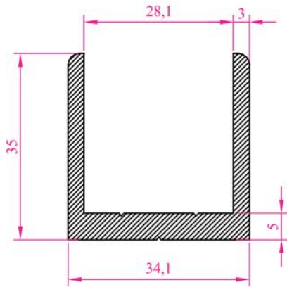
Profil No : 1016 Ag ırık : 0,943 kg/m
