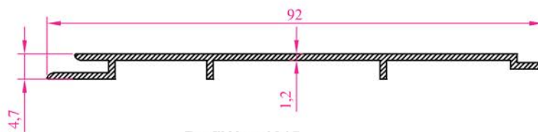
Profil N o : 1015 Ag ırık : 0,357 kg/m
