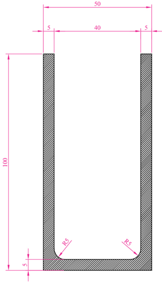
Profil No : 2806 Agırık : 3,281 kg/m
