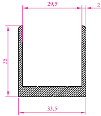
Profil N o : 2537 Ag ırık : 0,774 kg/m
