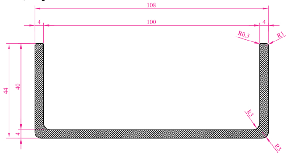
Profil No : 2839 Agırık : 2,037 kg/m
