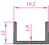
Profil N o : 2850 Ag ırık : 0,153 kg/m
