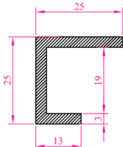
Profil N o : 2613 Ag ırık : 0,463 kg/m
