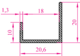
Profil N o : 2567 Ag ırık : 0,169 kg/m
