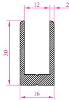
Profil N o : 2538 Ag ırık : 0,484 kg/m
