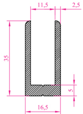
Profil N o : 1017 Ag ırık : 0,624 kg/m
