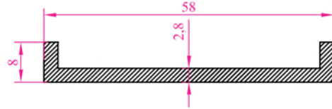
Profil No : 5158 Agırık : 0,519 kg/m
