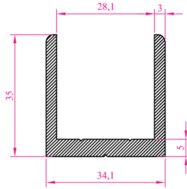
Profil N o : 1016 Ag ırık : 0,943 kg/m
